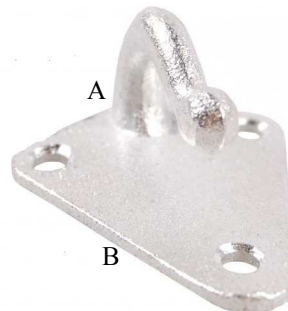
16-202-11 Driegats afdekhaak Vuurverzinkt Hoogte haak 25 mm en bij het laagste deel 19 mm. A: hoh 28 mm, totaal 40 mm B: hoh 32 mm, totaal 50 mm
